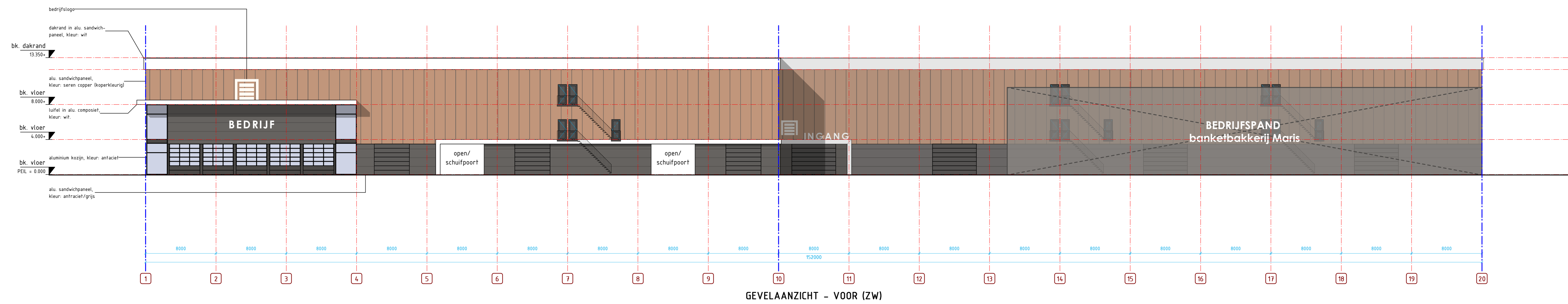
GEVELAANZICHT - VOOR (ZW)
